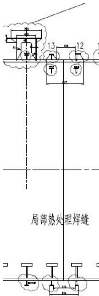
图 1-3 柱状壳带预焊件环缝示意图
