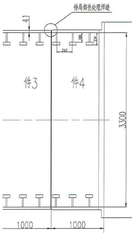
图 1-1 待局部热处理柱状壳体示意图
